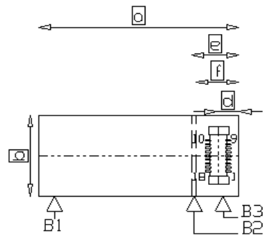
Vue de dessous, côté d'en fichage du connecteur
